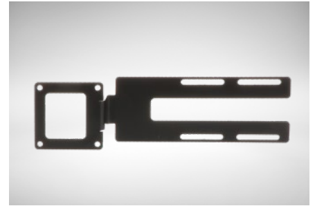
Montagekit für MFT1xSE seitliche Tastatur
